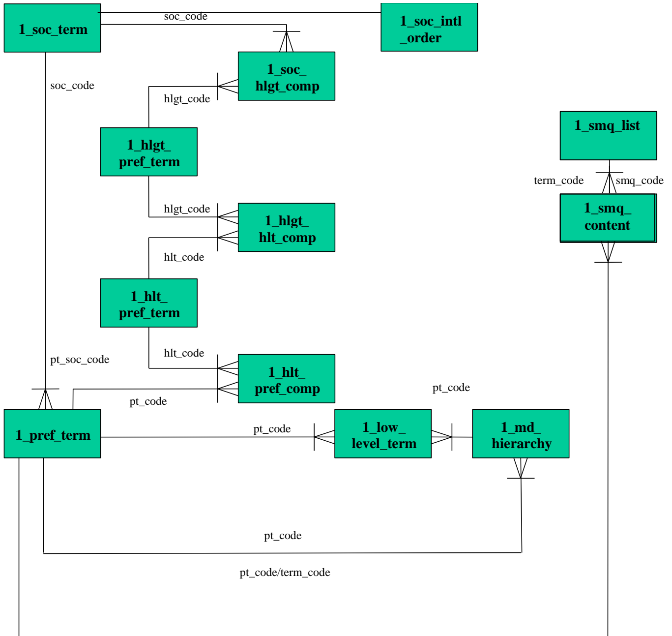
Abbildung 6-1. MedDRA Datenmodell
