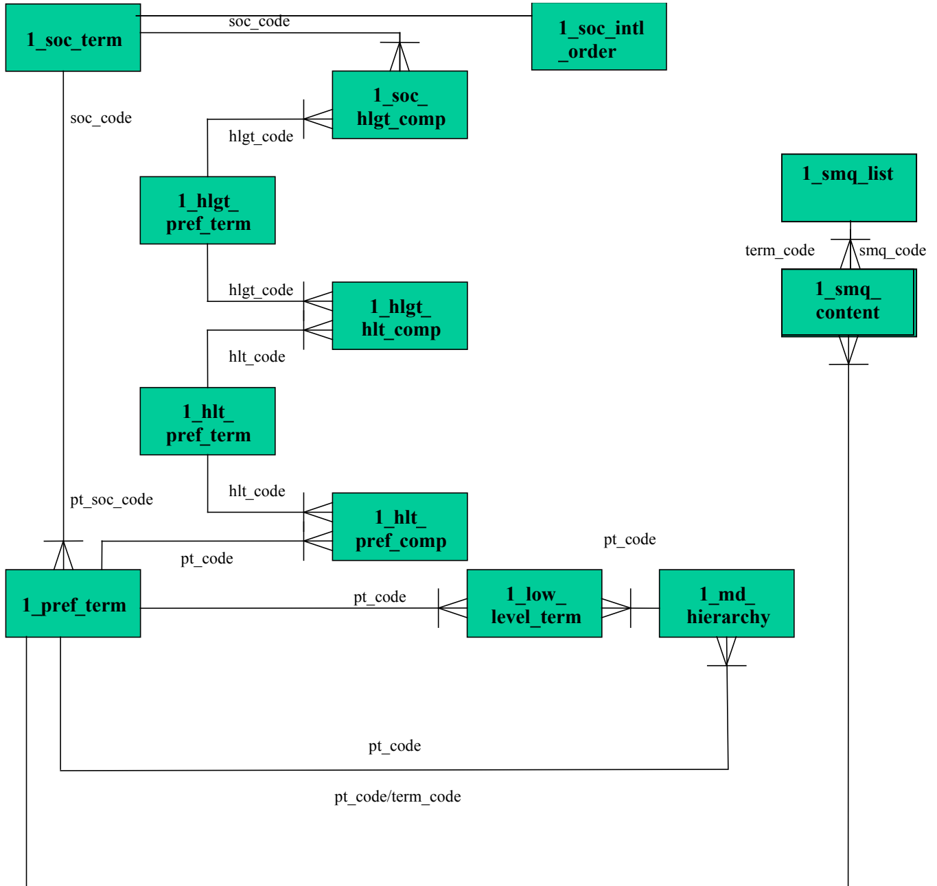
Abbildung 6-1. MedDRA Datenmodell
