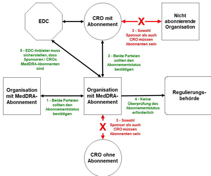
Abbildung 1 MedDRA-Austauschszzenarien
